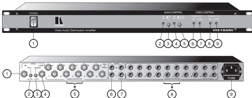
Рис. 2. Внешний вид передней и задней панелей VM-10ARII
