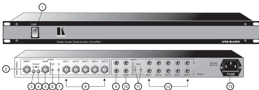
Рис. 1. Внешний вид передней и задней панелей VM-5ARII
